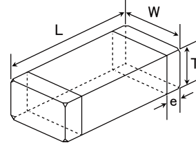
5面電極
